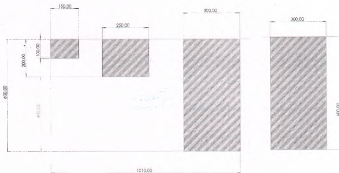
Сурет-1 микро доғалық тотығуға арналған ванна схемасы (бірлік. миллиметрмен)
